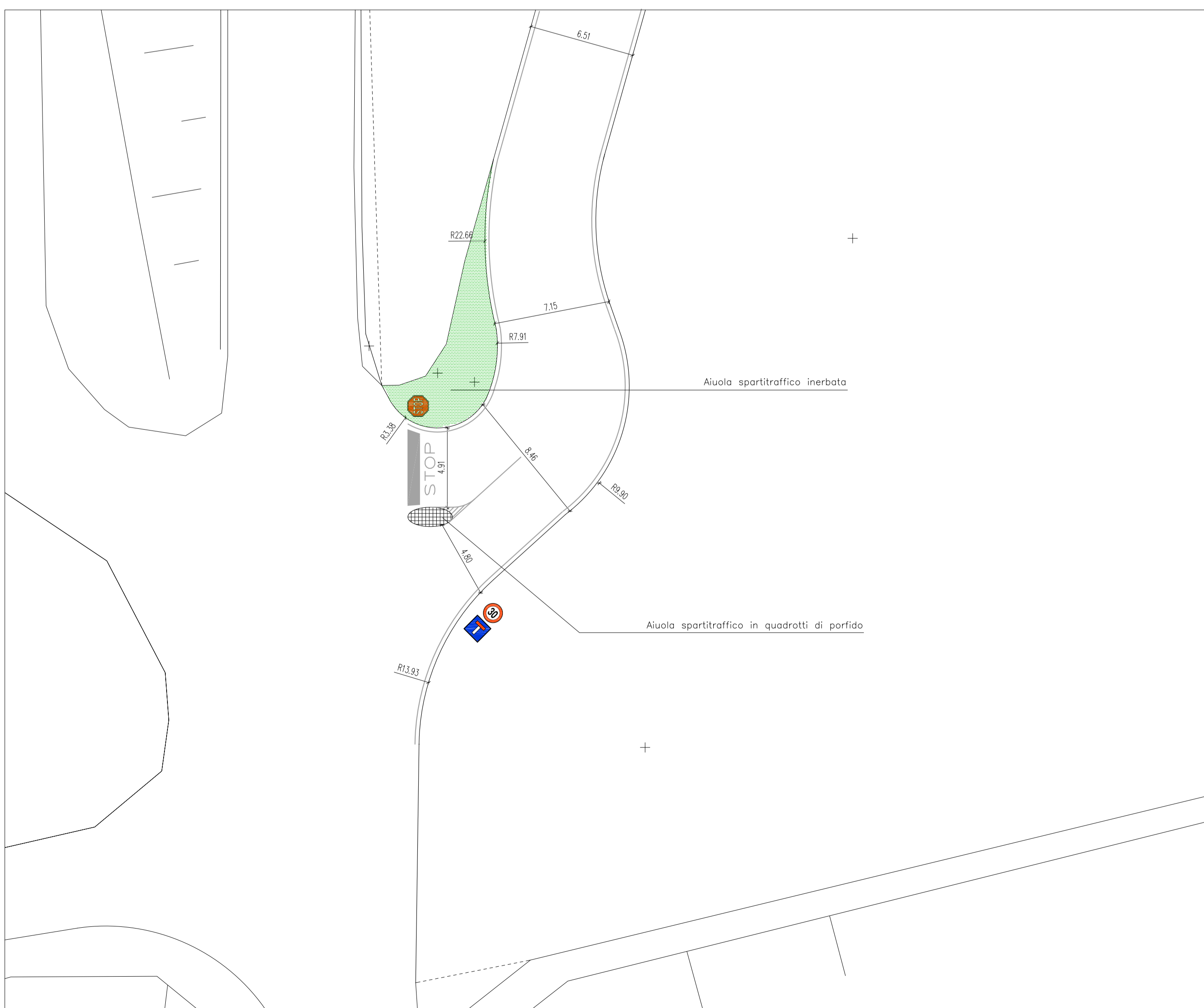
Nuova intersezione con la Strada Provinciale Segnaletica orizzontale e verticale
