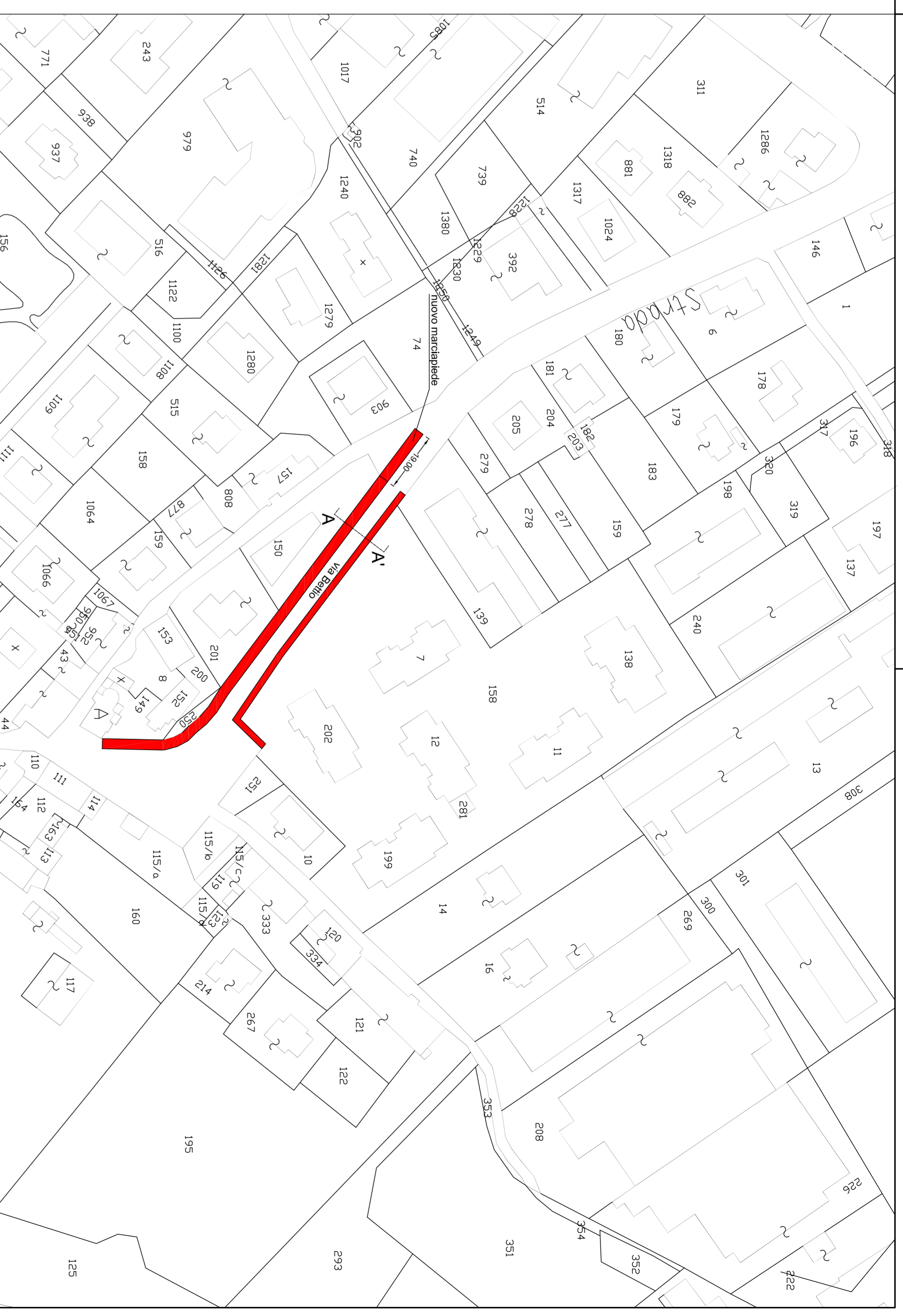
PLANIMETRIA SCALA 1:1000
