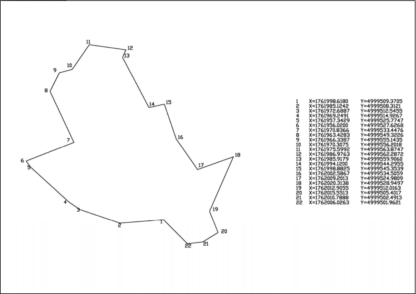
COORDINATE DEI VERTICI (GAUSS-BOAGA OVEST)
