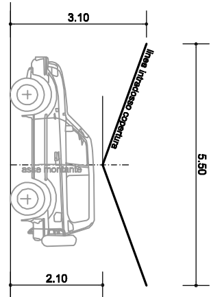
TETTOIA SU PALI LEGNO O ACCIAIO
