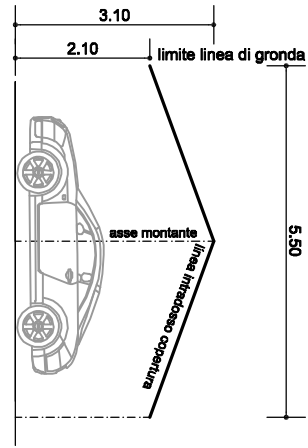
TETTOIA SU PALI SOLO RIFINITURE IN LEGNO (solo in tegole simitopoli)
