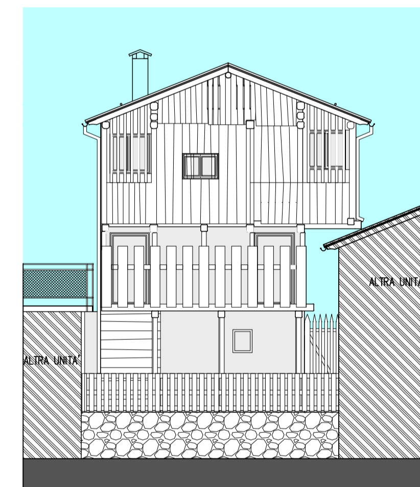
Prospetto OVEST
