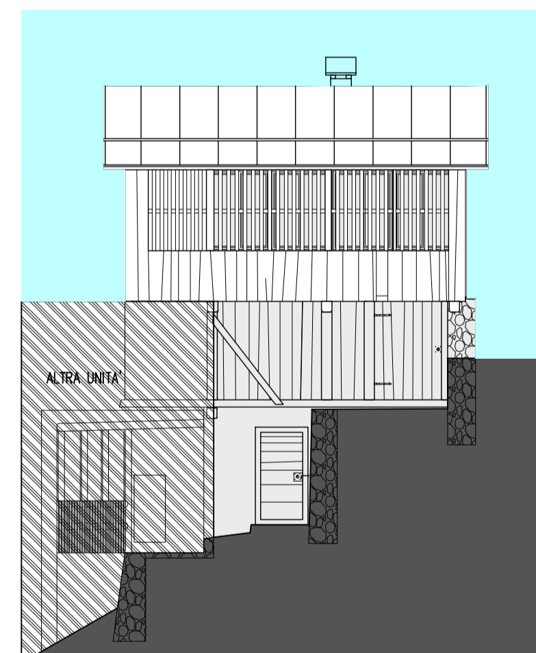
Prospetto SUD
