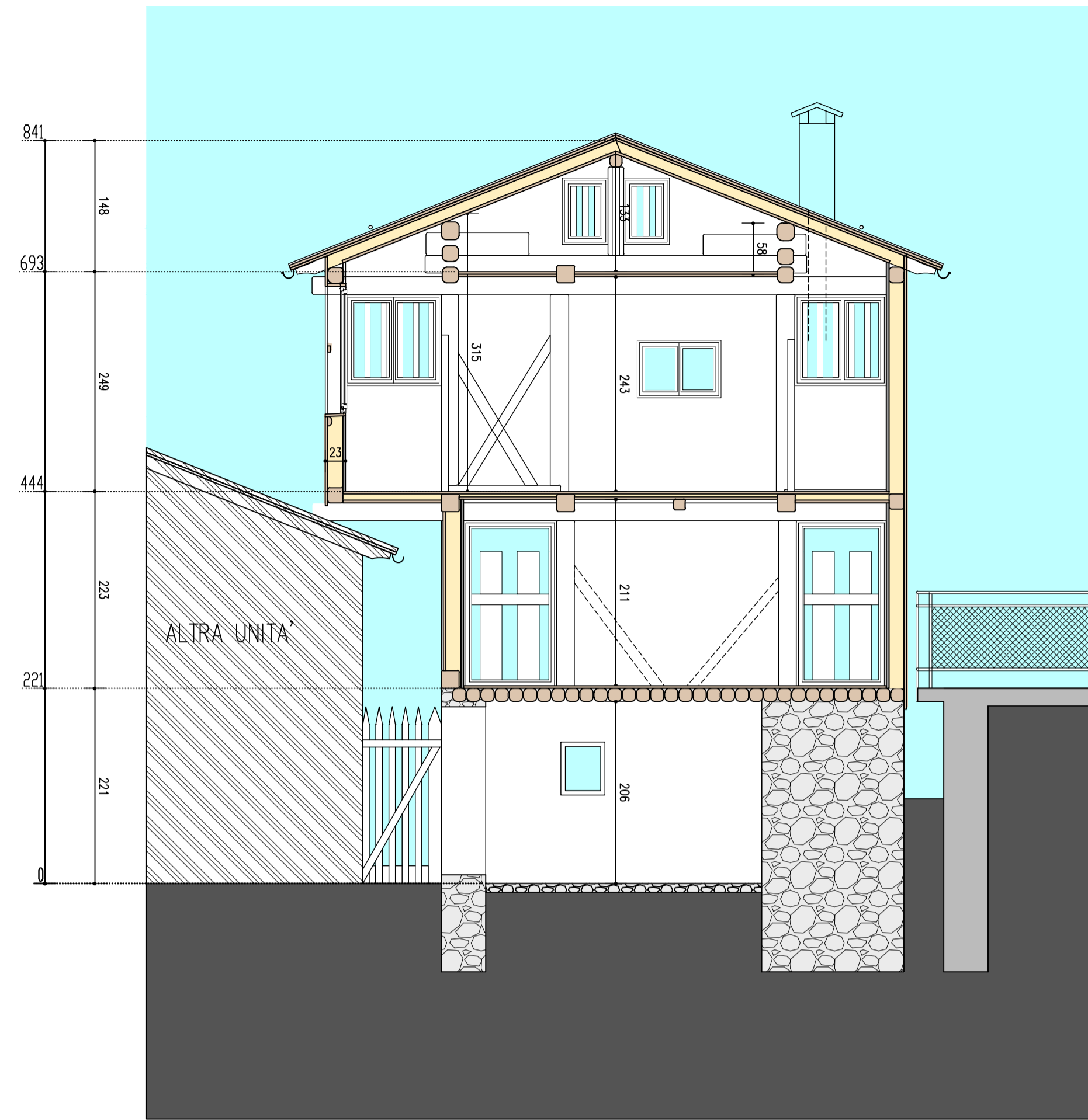
Sezione A-A
